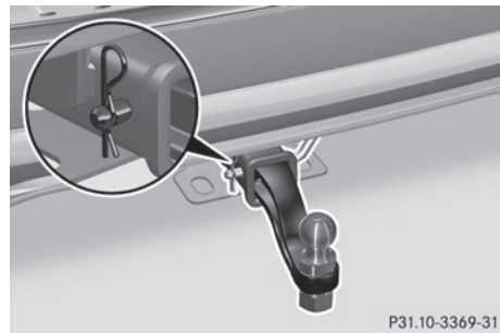
Pose et verrouillage corrects de la rotule
